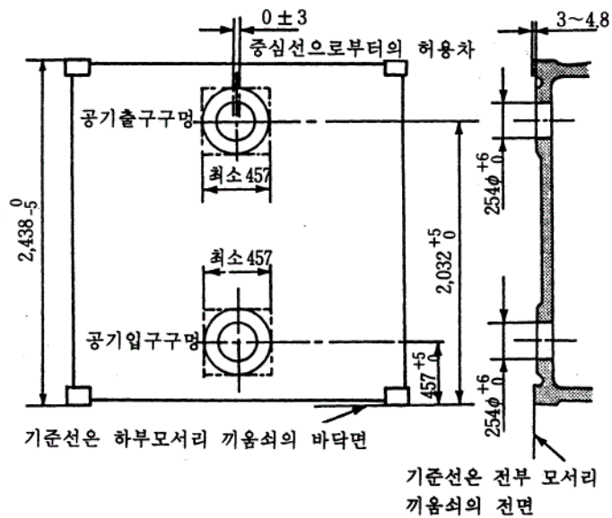
그림 2.20 1C 방열 컨테이너 단부벽의 공기구멍
