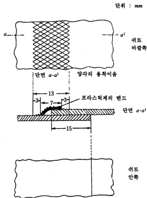
그림 4 여러 조각으로 만들어진 시트의 융착에
