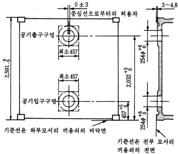
그림 2.19 1CC 방열 컨테이너 단부벽의 공기구멍
