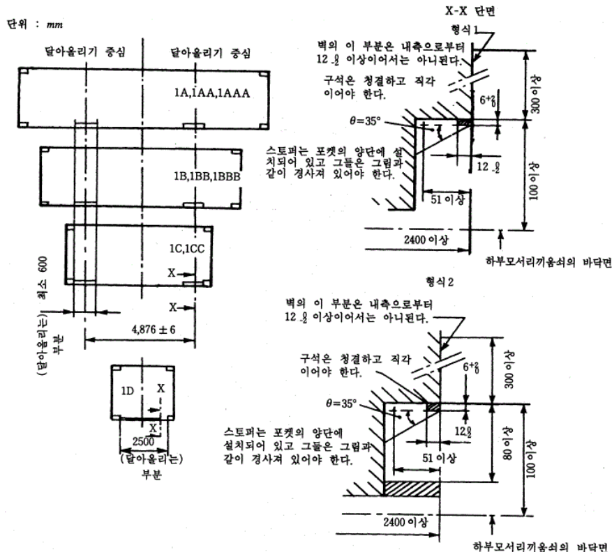
그림 2.15 그레플 암의 갈고리 구조
