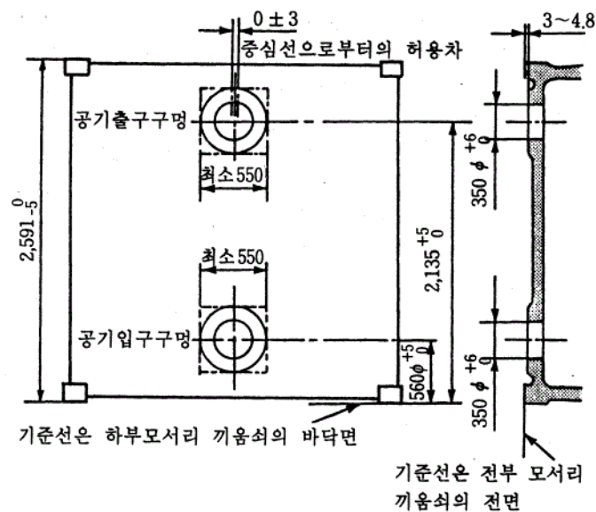
그림 2.18 1AA 방열 컨테이너 단부벽의 공기구멍
